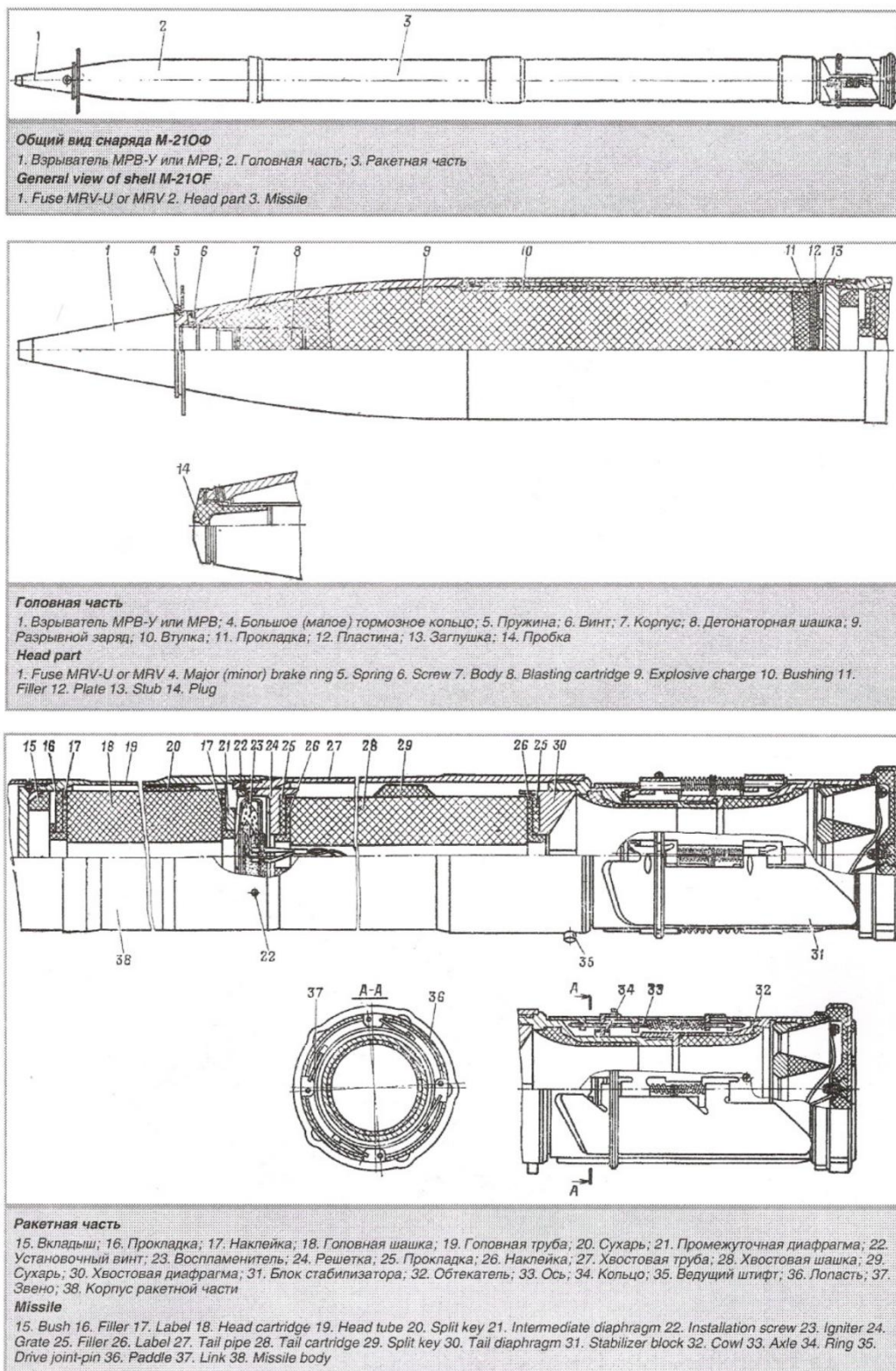
Рисунок 22. Конструкция снаряда М-210Ф (осколочно-фугасный снаряд, применяемый для стрельбы из РСЗО БМ-21 «Град»). 19
